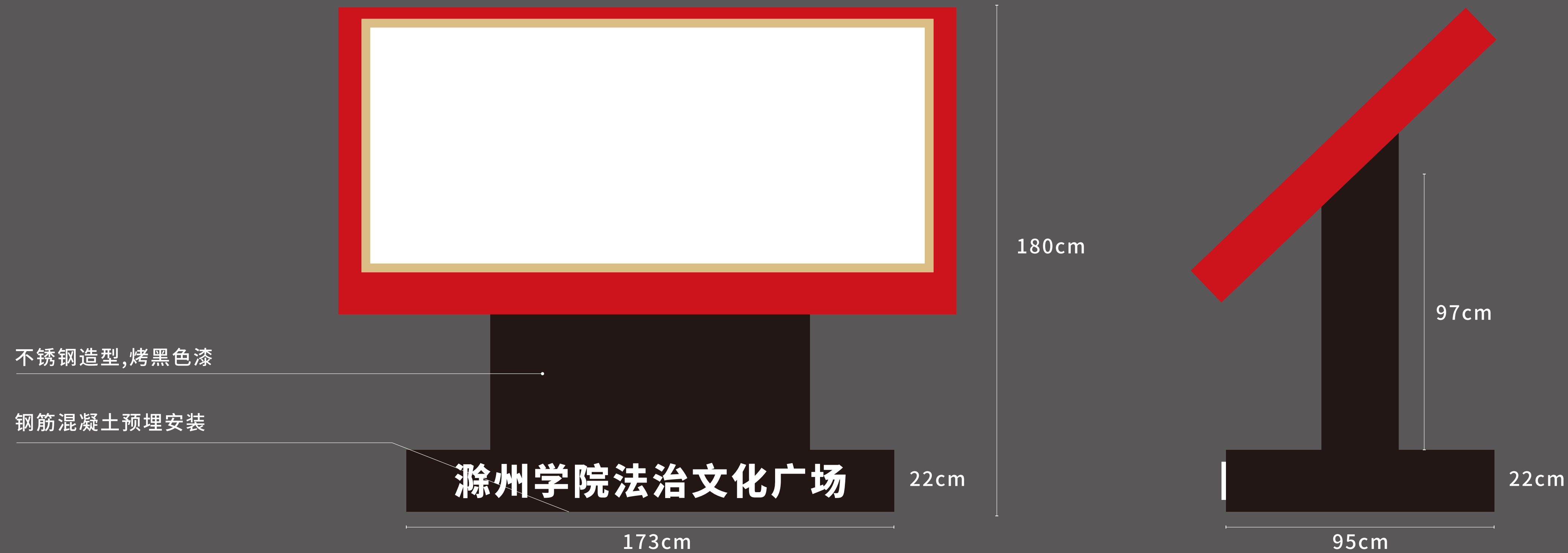
正视图
